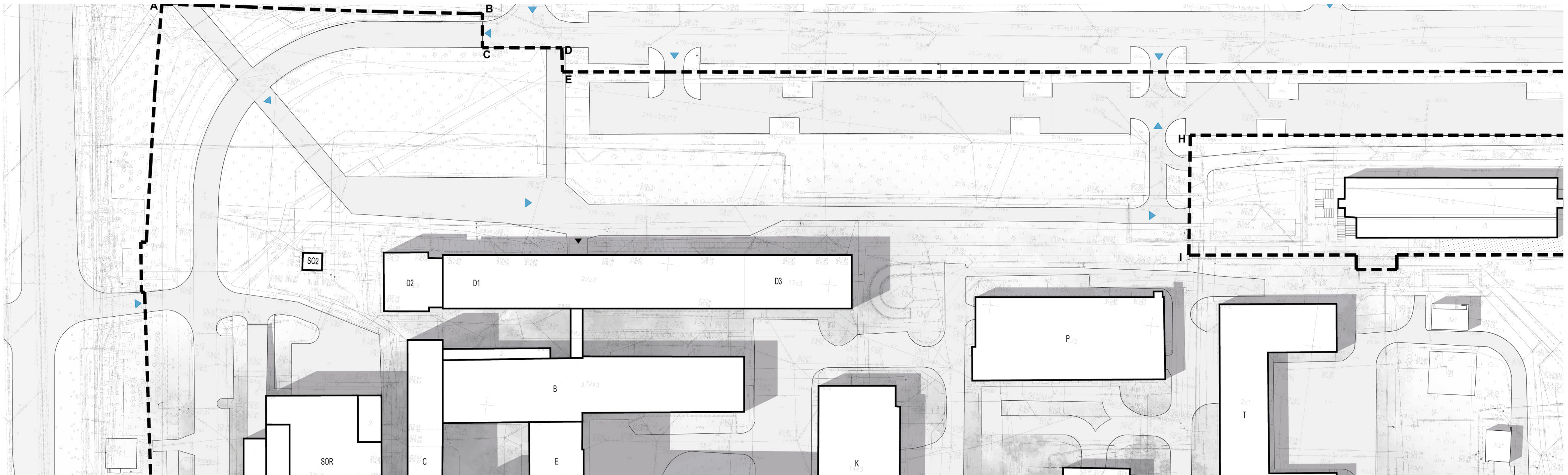
ZAGOSPODAROWANIE TERENU SKALA 1:500
